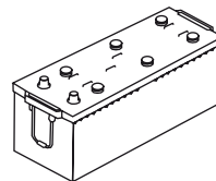
A + - 513x189x194/220 63530
