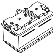
L5 - + 353x175x190 58822
